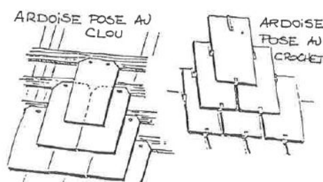
POSE DES ARDOISES
