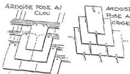
POSE DES ARDOISES
