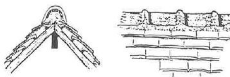
CRETES ET EMBARRURES DES PATAGES DE TERRE CUITE SANS EMBOITURE
