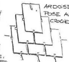
POSE DES ARDOISES
